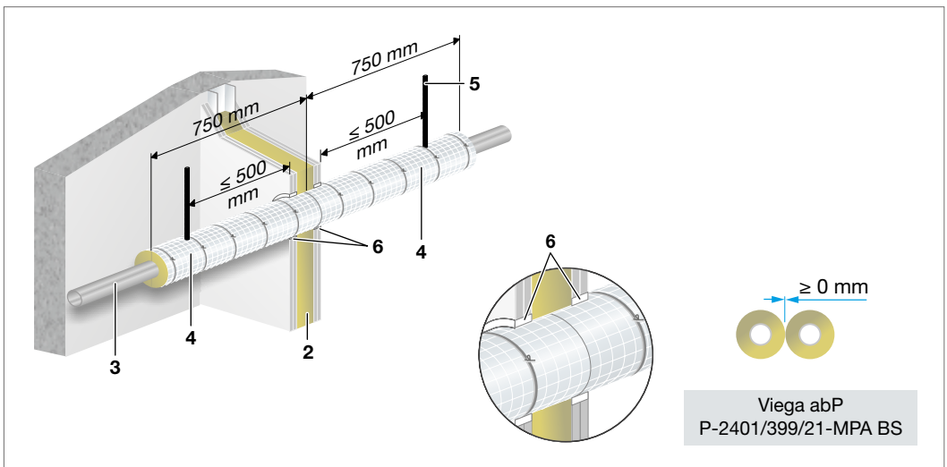
Abb. 159: Prestabo/Prestabo PP-ummantelt – Einbau in leichte Trennwand
