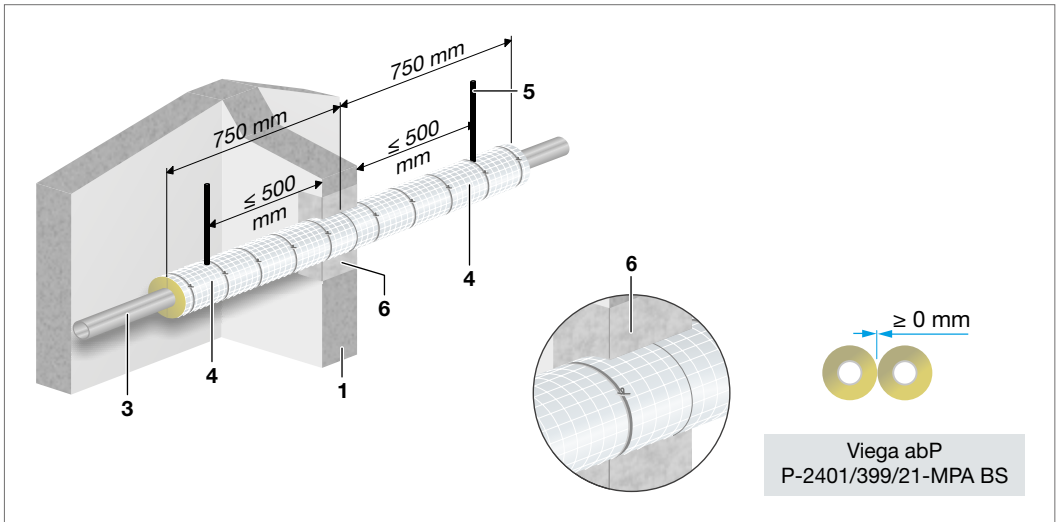
Abb. 158: Prestabo/Presstabo PP – Einbau in Massivwand
