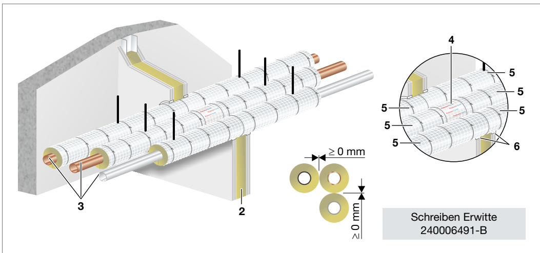
Abb. 171: Viega Metallrohrsysteme im Nullabstand Rockwool Conlit 150U abP P-3725/4130-MPA-BS – leichte Trennwand
