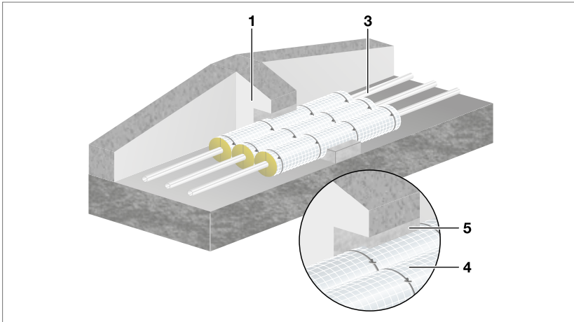
Abb. 187: Wandschließung mit Sanfix Fosta/Raxofix durch Massivwand, R 30/R 60/R 90
