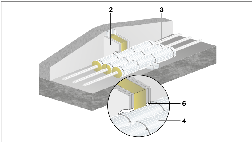
Abb. 188: Wandschließung mit Sanfix Fosta/Raxofix durch leichte Trennwand, R 30/R 60/R 90
