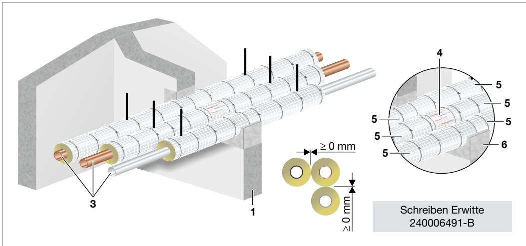
Abb. 170: Viega Metallrohrsysteme im Nullabstand Rockwool Conlit 150U abP-3725/4130-MPA-BS – Massivwand
