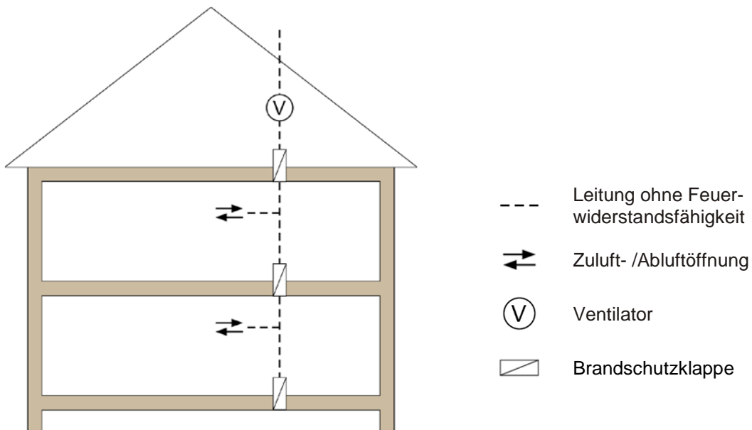
Bild 2.1: Schottlösung
