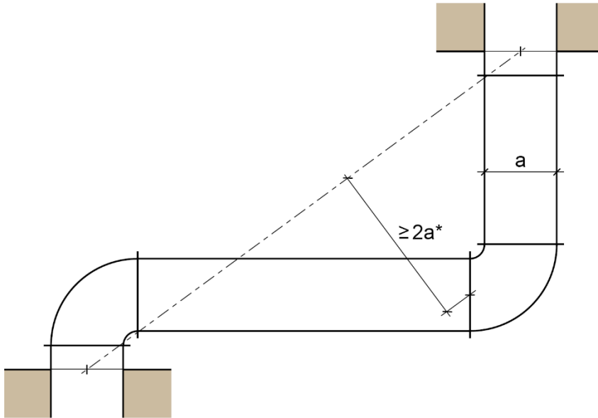
Bild 5.1: Begrenzung der Krafteinleitung mit Leitungsverzierung
