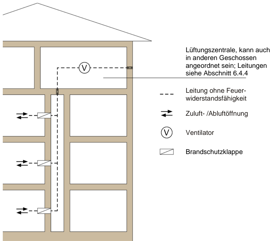
Bild 1.2: Schachtlösung Brandschutzklappen an den Durchdringungsstellen der feuerwiderstandsfähigen Schachtwände
