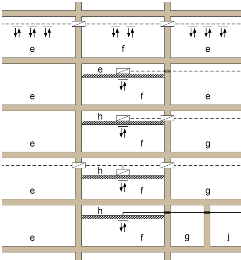
Bild 3.2: notwendiger Flur belüftet
