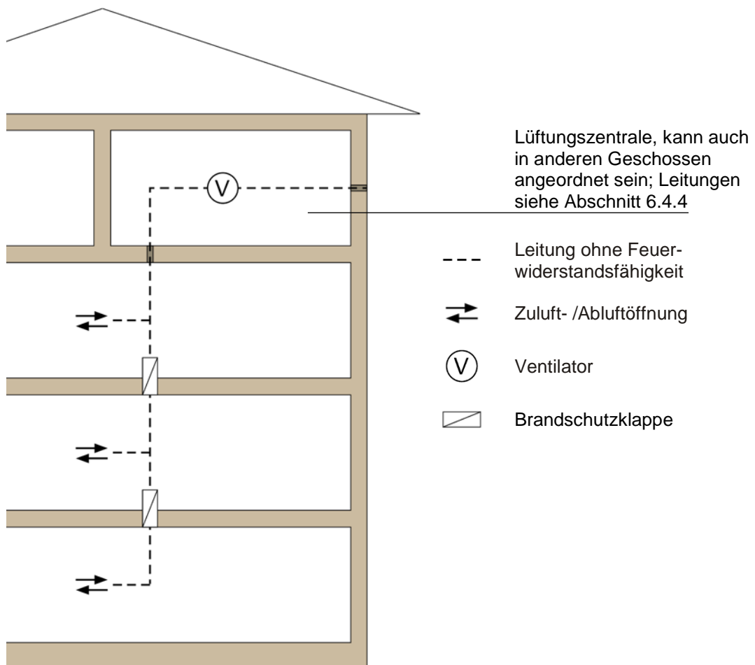
Bild 1.1: Schottlösung Brandschutzklappen an den Durchdringungsstellen der feuerwiderstandsfähigen Decken
