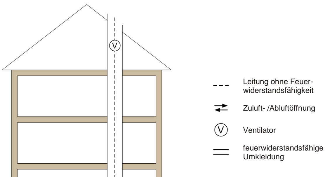
Bild 2.2: Schachtlösung
